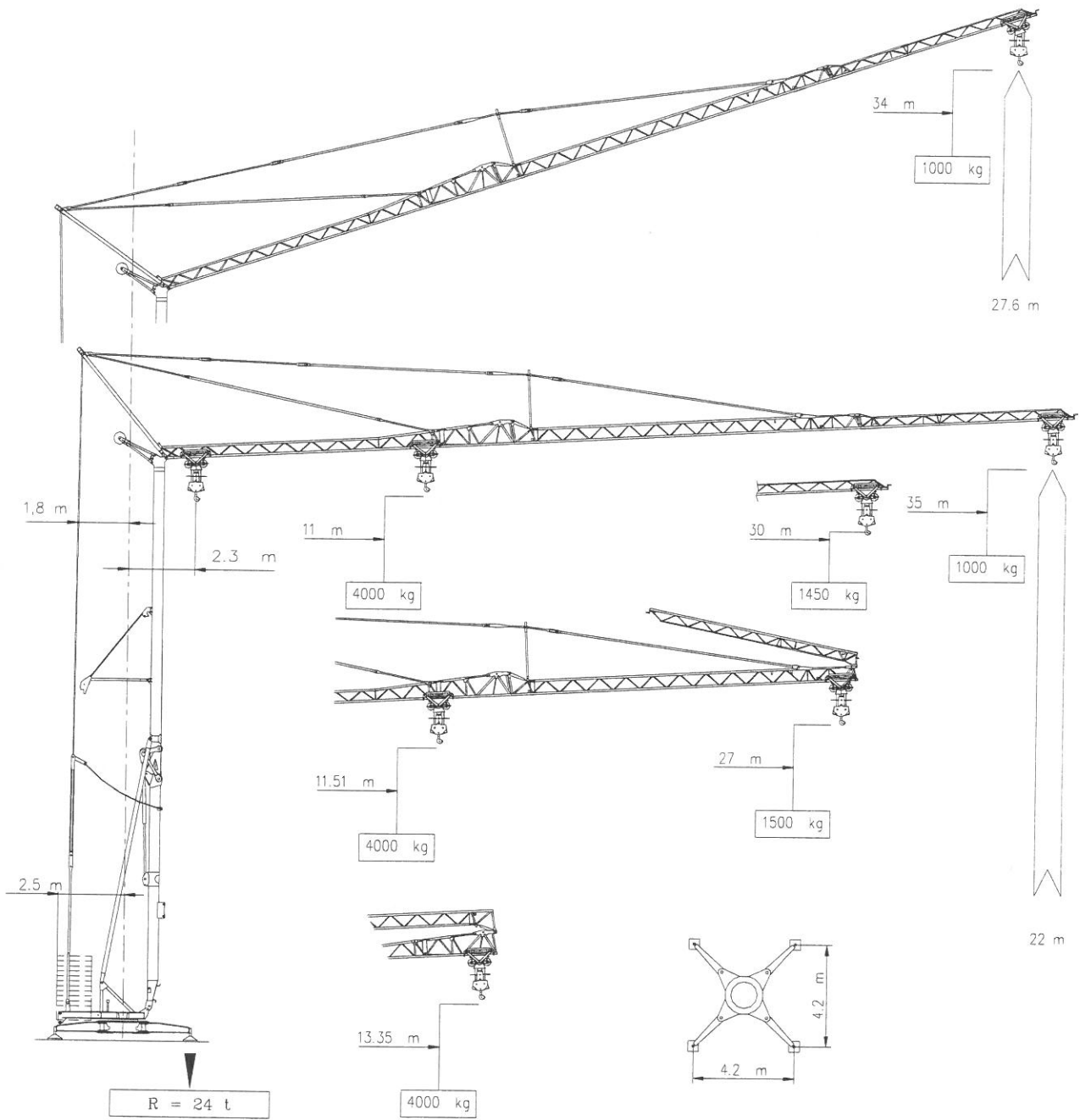
LOAD CURVES - LASTKURVEN - COURBES DE CHARGES - CURVE DI CARICO - CURVAS DE CARGA
